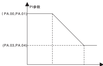
图8-23 PI参数示意图
