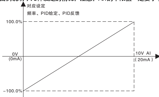
图8-13 模拟给定与设定量的对应关系
