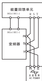
图6-14 能量回馈单元连接图
