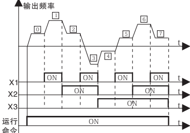
图8-22 多段速度运行逻辑图
