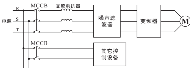
图6-12 主回路电源侧连接图
