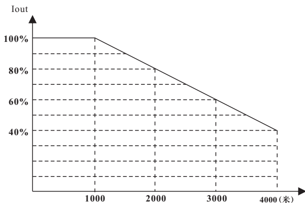
图3-1 安装地点的海拔高度
