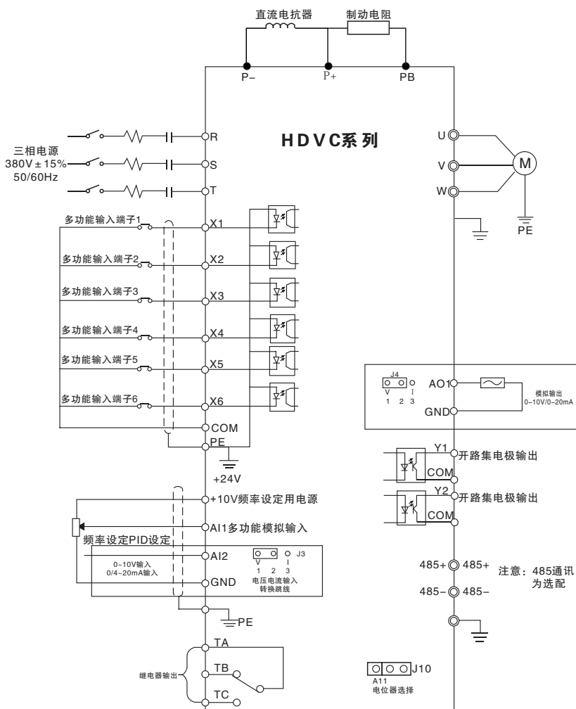
图4-11 标准接线图
