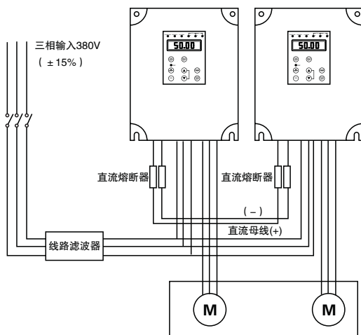
图6-15 共直流母线的连接
