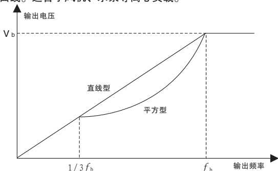
图8-3 V/F曲线示意图
