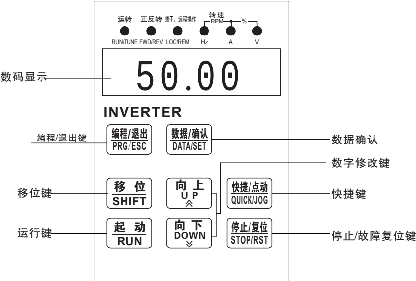
图7-1操作面板示意图
