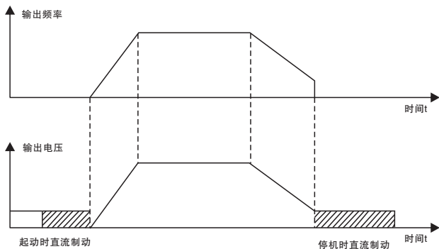
图8-6 直流制动示意图
