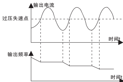
图8-15 过压失速功能
