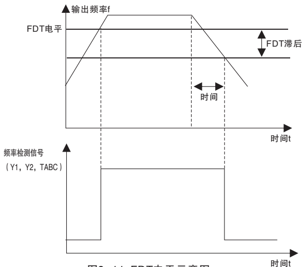
图8-11 FDT电平示意图
