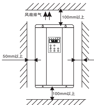
图3-2 安装的间隔距离
