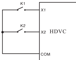
图8-8 两线式运转模式2示意图
