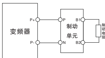
图10-2 制动单元的连接
