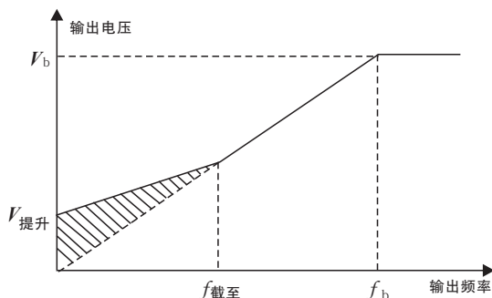
图8-4 手动转矩提升示意图
