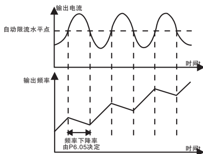
图8-17 限流保护功能示意图
