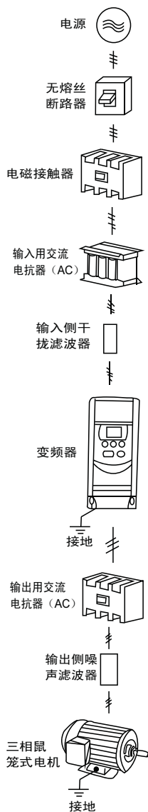
图4-1 外围设备的连接图
