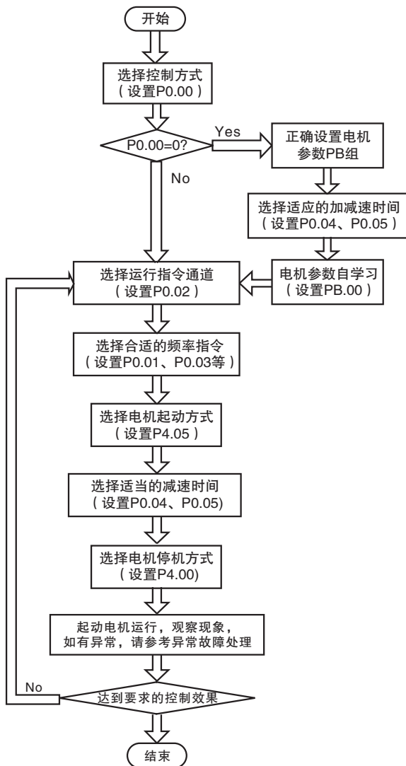
图7-3 快速调试流程图
