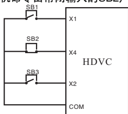
图8-10 三线式运转模式2示意图
