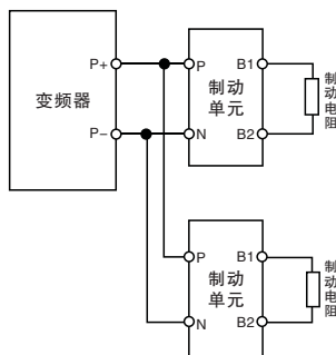
图10-3 制动单元的并联连接
