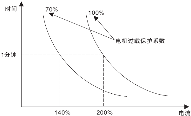
图8-16 电机过载保护系数设定
