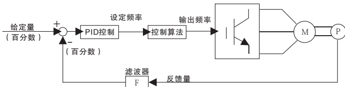
图8-20 过程PID原理框图
