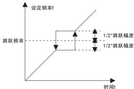
图8-18 跳跃频率示意图
