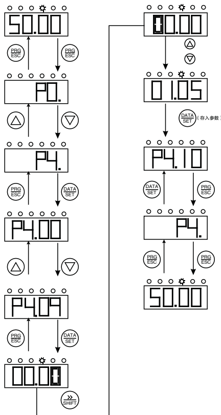
图5-2 三级菜单操作流程图
