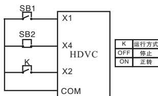
图8-9 三线式运转模式1示意图
