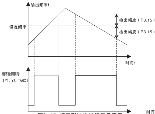
图8-12 频率到达检出幅值示意图
