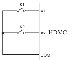
图8-7 两线式运转模式1示意图
