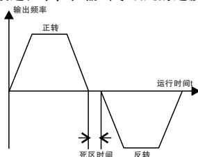
图8-5 正反转死区时间示意图
